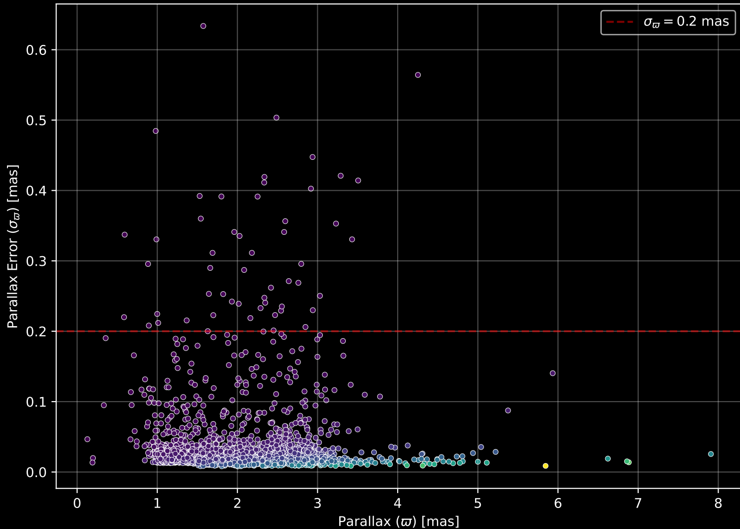
GALAH DR4 Field: [-8] Parallax Quality (n= 4043)
