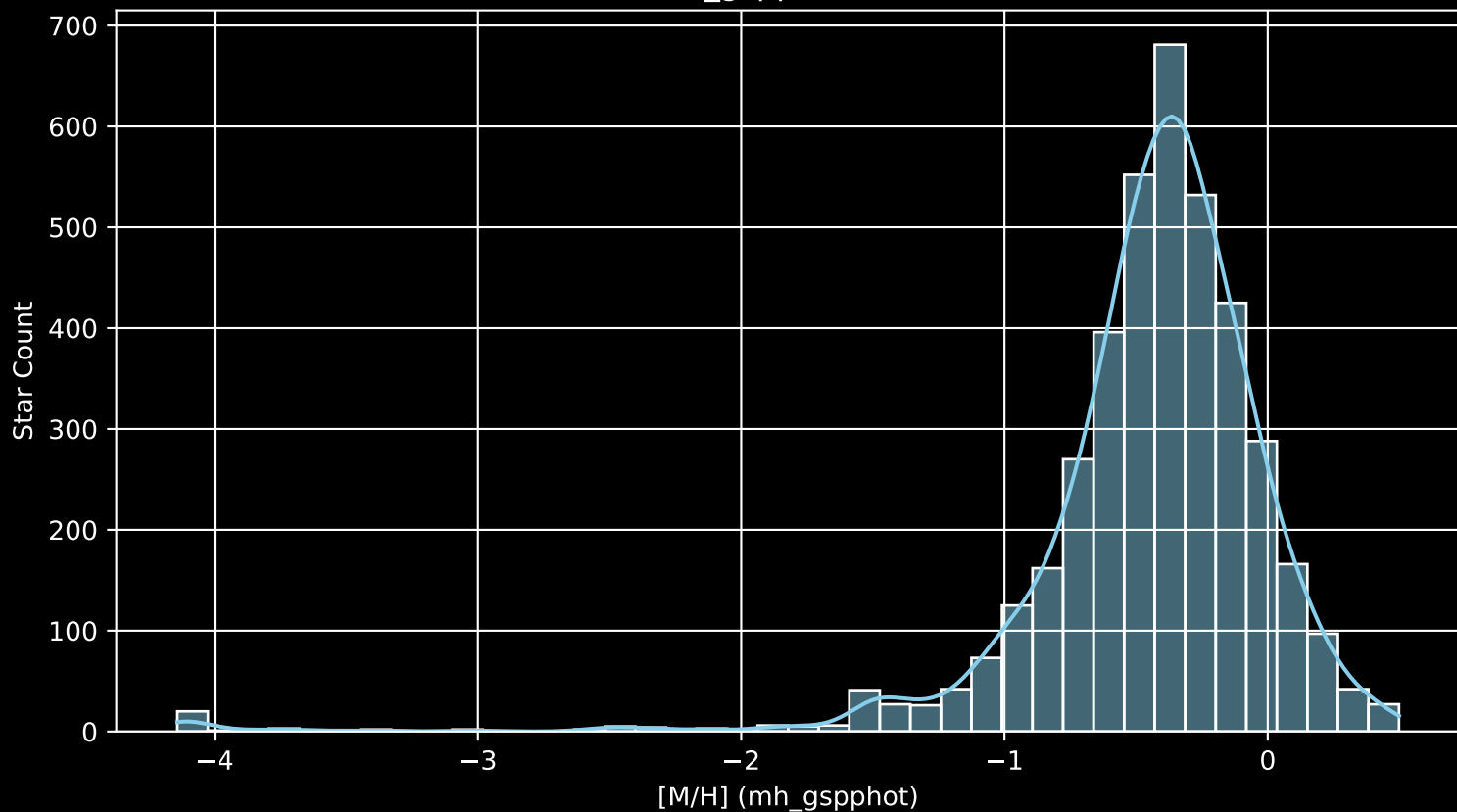
GALAH DR4 Field: [-8] [M/H] (mh_gspphot) (n= 4036)
