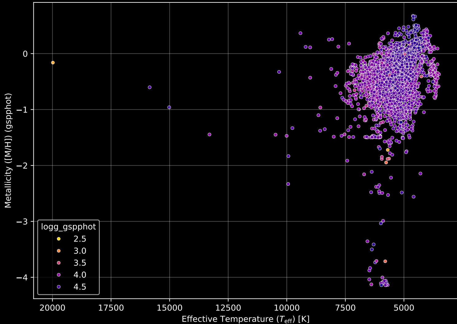
GALAH DR4 Field: [-8] Stellar Population Parameters (n= 4043)
